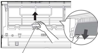
Zatiči filtra
